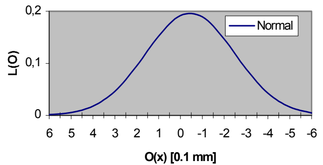
Fig. 12 Täthetsfunktion för bockning med rits
